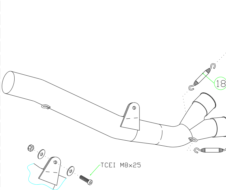
71310MI Raccordo basso / Low Mid Pipe
