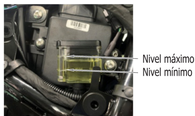
Líquido de frenos trasero
