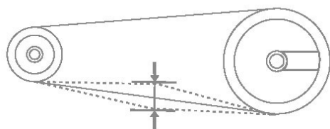
Holgura o juego libre de la cadena: 18-25 mm
