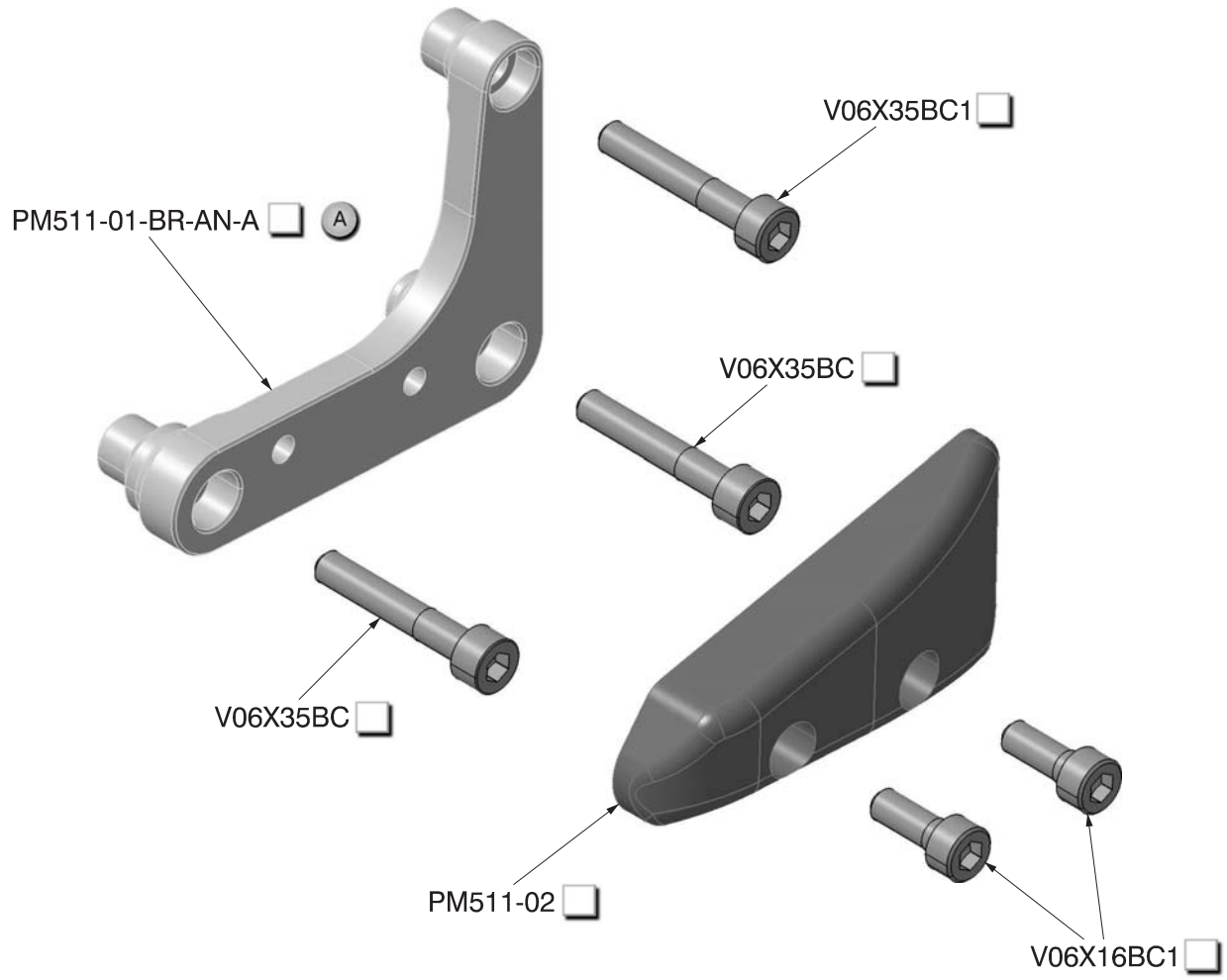
PM511 (Protezione coperchio impuls completa) A (Complete crankcase guard)
