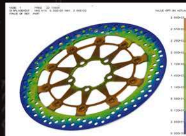
>Analisis de esfuerzos / Stress Simulation
