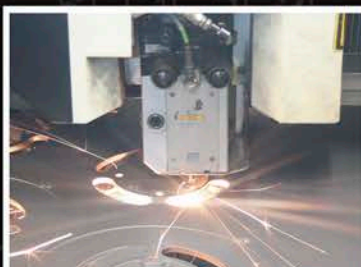
>Laser / Laser cut
