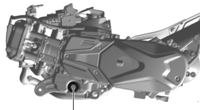
Tornillo tamiz filtro de aceite
