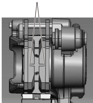
Límite de desgaste de las pastillas traseras
