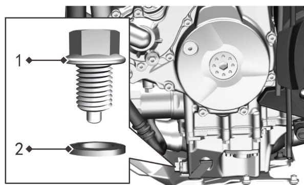
1: Tornillo de drenaje 2: Junta
