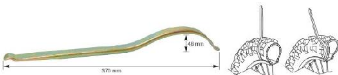
Ref. 19384 Desmontable de cubiertas curvo. 370 mm Para cubiertas tipo "balón" y "todoterreno" Cromoly. 400g.
