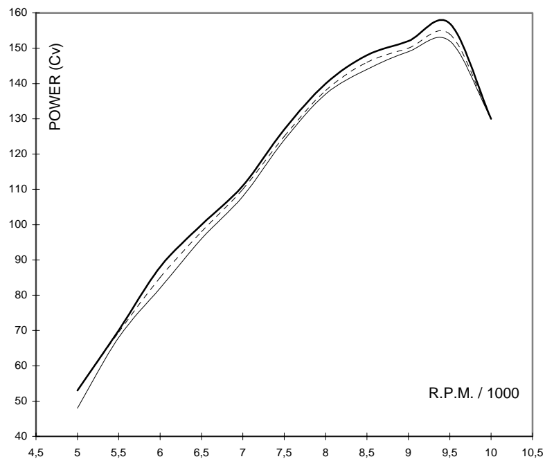
Power chart / Leistungsschaubild Graphique de puissance / Grafica de potencia
