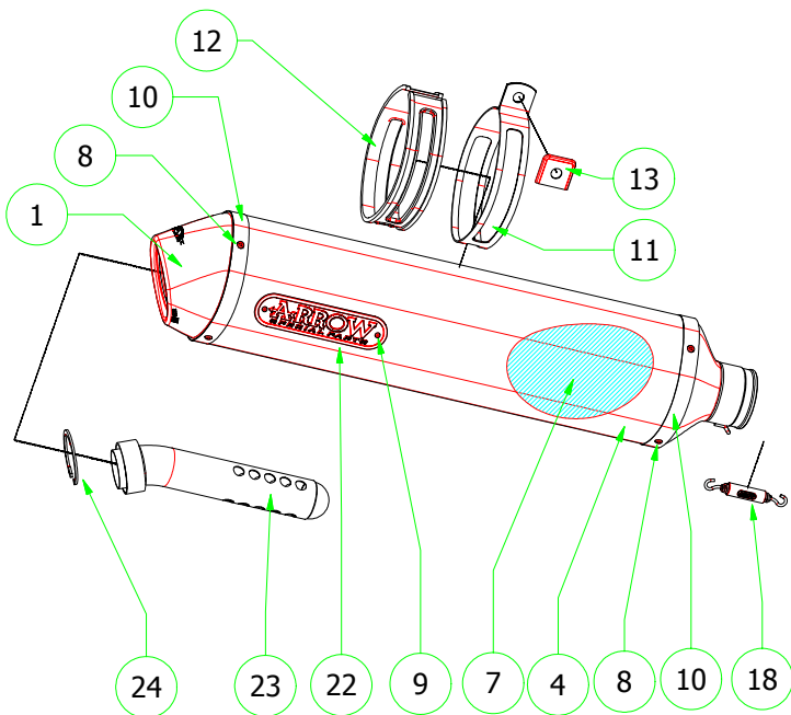
71234MI Raccordo Basso Low Mid Pipe
