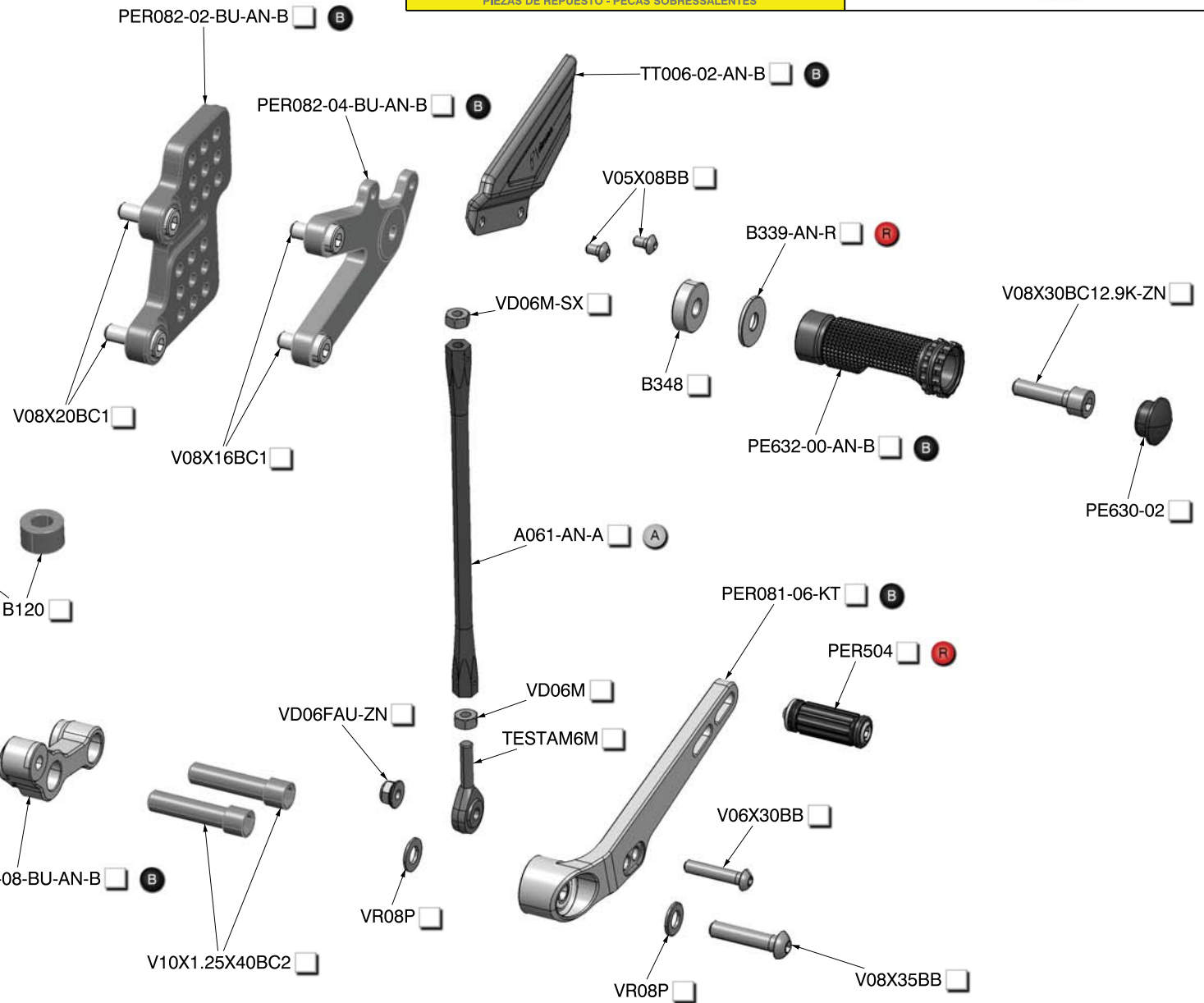
PER082-SX (Comandi arretrati lato SX completi) (Complete LH rear set control kit)
