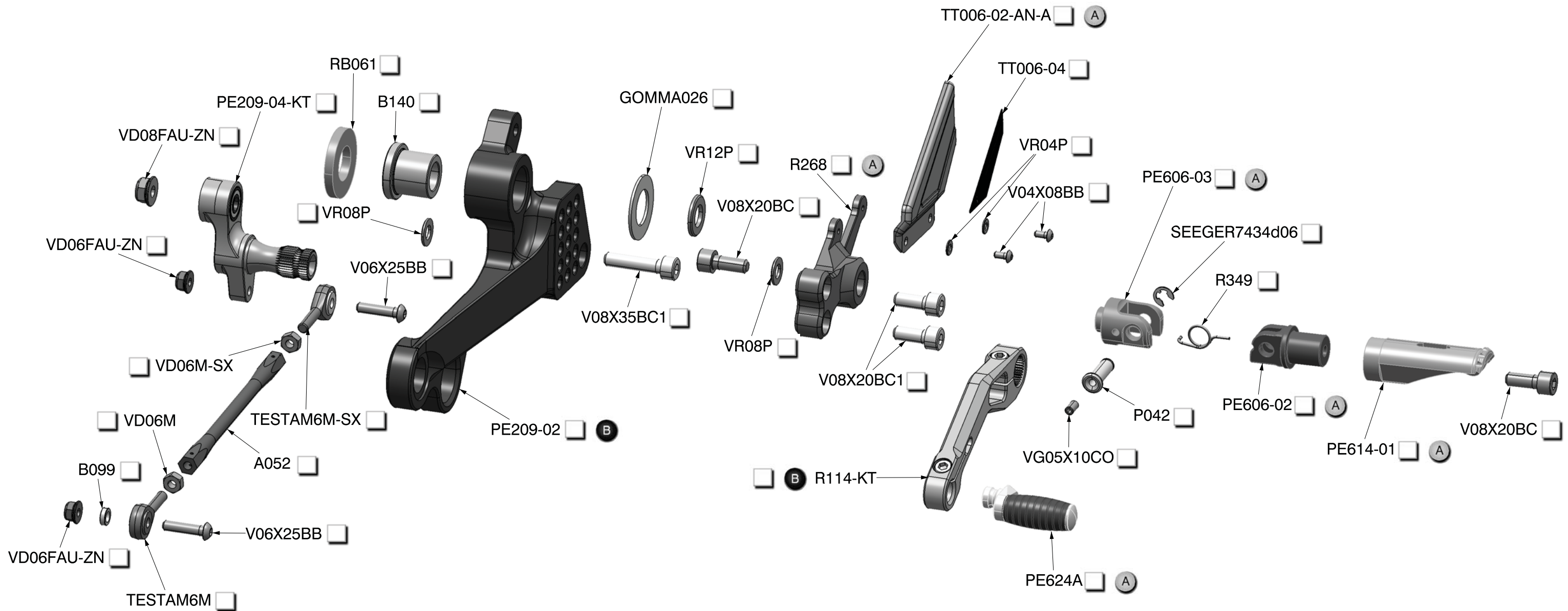
PE209-SX (Comandi arretrati lato SX completi) B (Complete LH rear set control kit)
